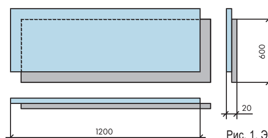
Рис. 1. Элемент пола
